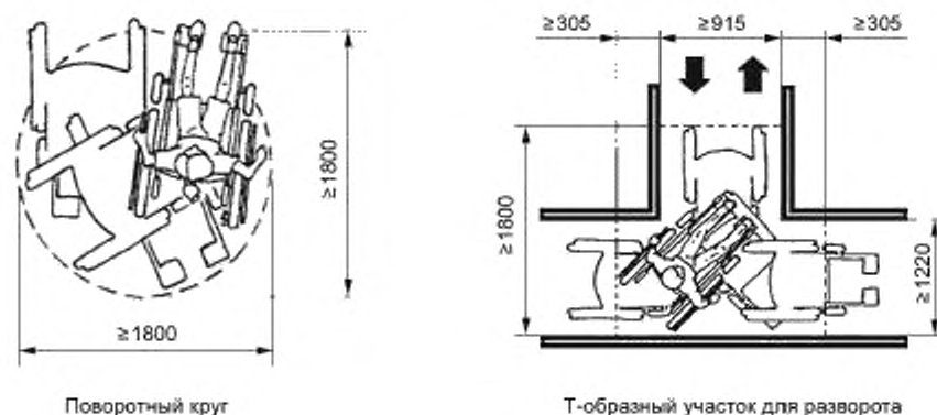
Рисунок 2 — Устройство поворотного круга и Т-образного участка
