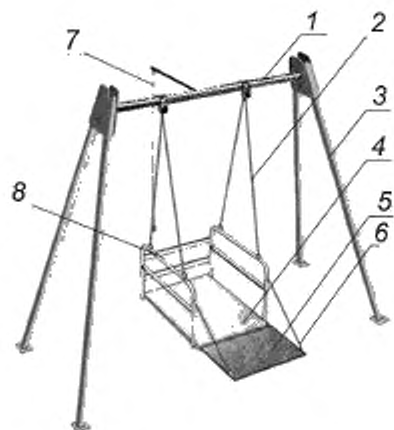
1 — балка; 2 — цепь; 3 — стойка; 4 — платформа качелей для кресла-коляски; 5 — откидной пандус; 6 — цепь крепления откидного пандуса; 7 — устройство самораскачивания; 8 — ограждение платформы качелей
