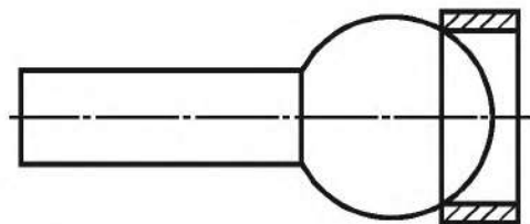
Рисунок Г.2 — Допустимый вариант торцевой части рукоятки
