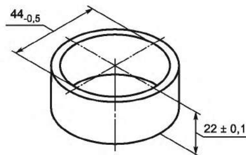
Рисунок Г.1 — Калибр
