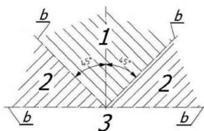
б) Расположение зон по отношению к вертикальной и горизонтальной осям 1 – зона 1; 2 – зона 2; 3 – зона 3
